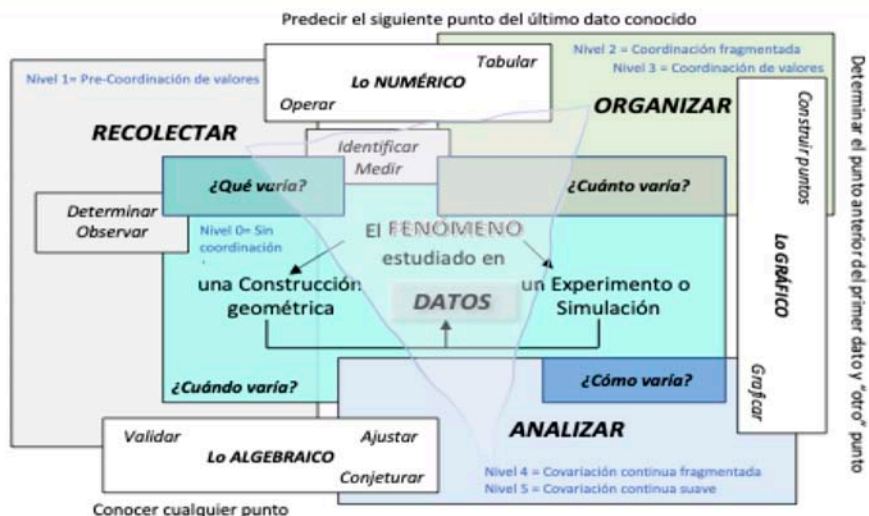
FIGURA 2. Modelación-covariación logarítmica-exponencial
