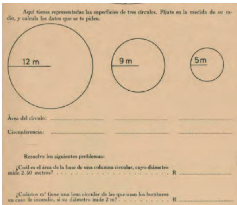
FIGURA 1. Área de círculos
