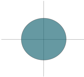
Figura 1.3: 2-bola cerrada.
