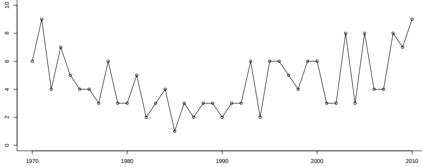
Figura 3.1: Número de ciclones que han impactado a México
