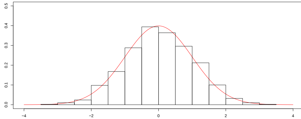
Figura 3.9: Distribución de Z
