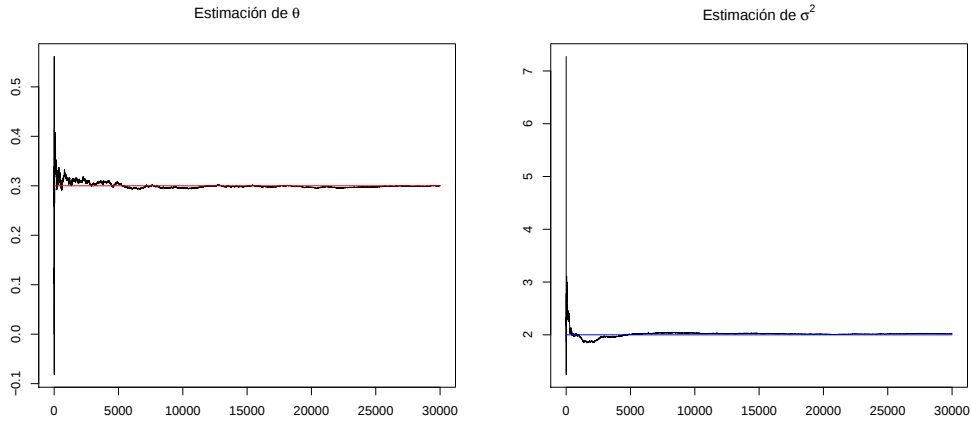
Figura 3.8: Estimación de los parámetros
