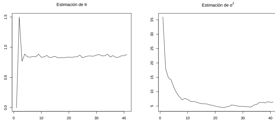
Figura 3.2: Estimación de los parámetros
