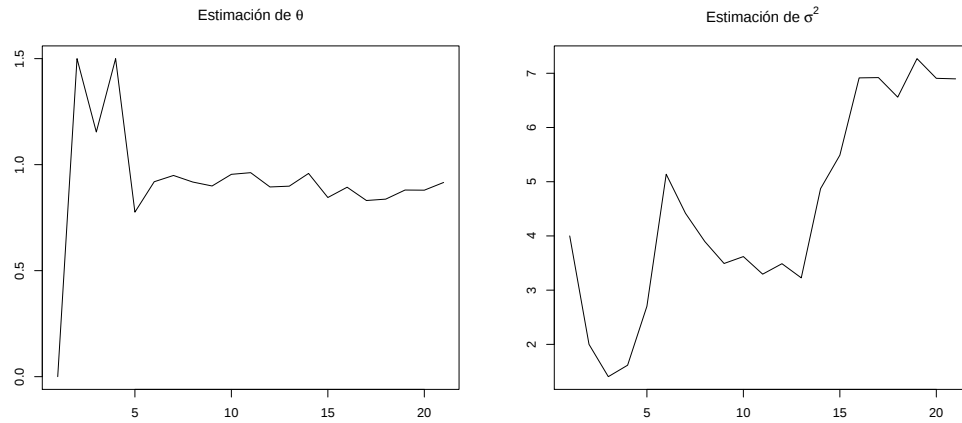
Figura 3.2: Estimación de los parámetros
