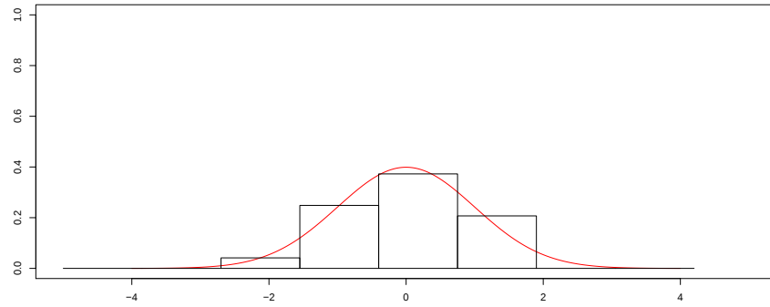
Figura 3.4: Distribución de los residuos
