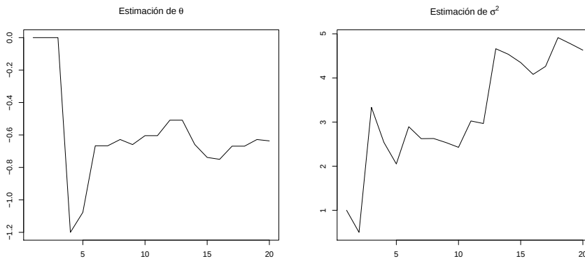
Figura 3.6: Estimación de los parámetros con Primeras Diferencias
