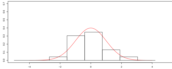
Figura 3.7: Distribución de los residuos con Primeras Diferencias
